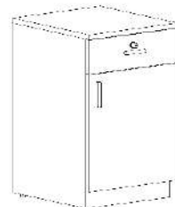
1 Drawer Shutter Pedestal Unit 405 X 450 X625 - UM-OPUES03 405 X 450 X650 - UM-OPUES04
